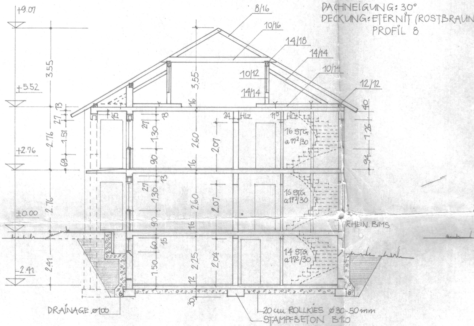
SCHNITT A-A
